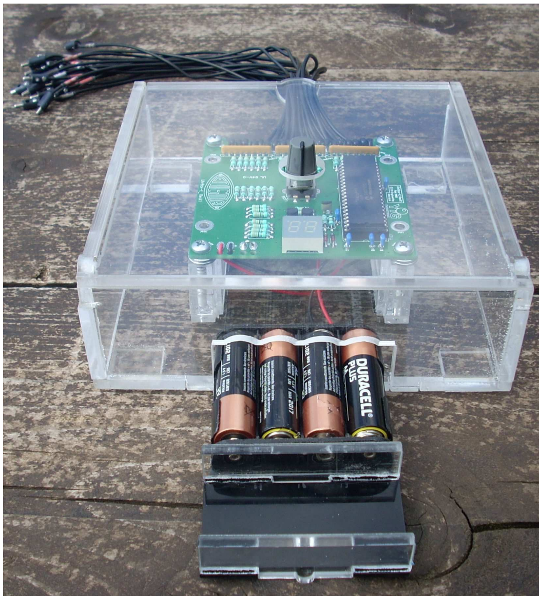
Rear view with battery box open. Vista posteriore col vano batterie aperto.
