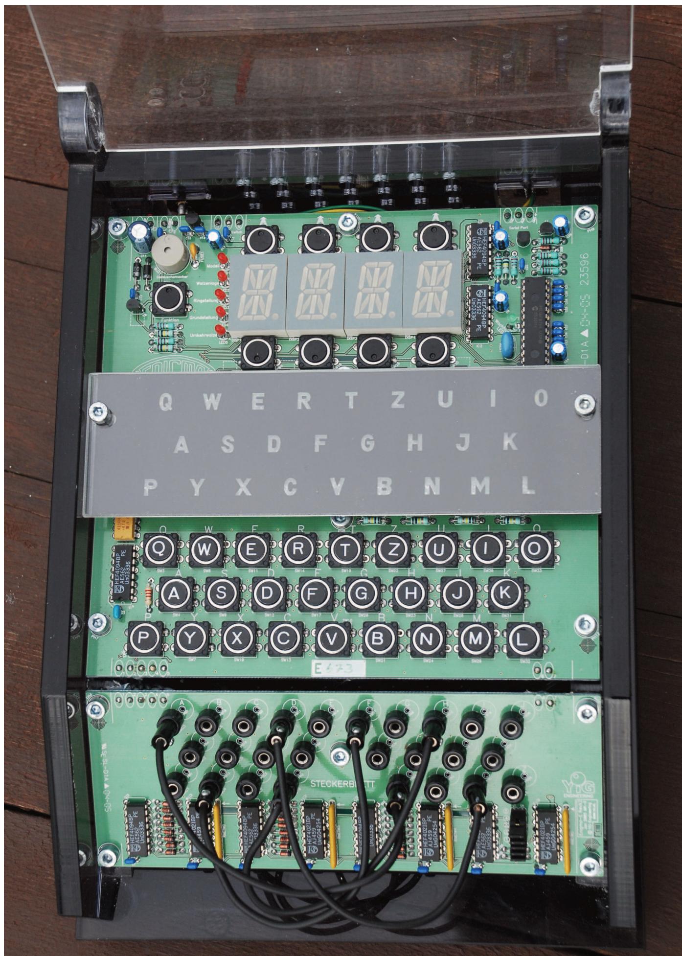
Vista dall'alto col coperchio alzato - Top view with lid open.
